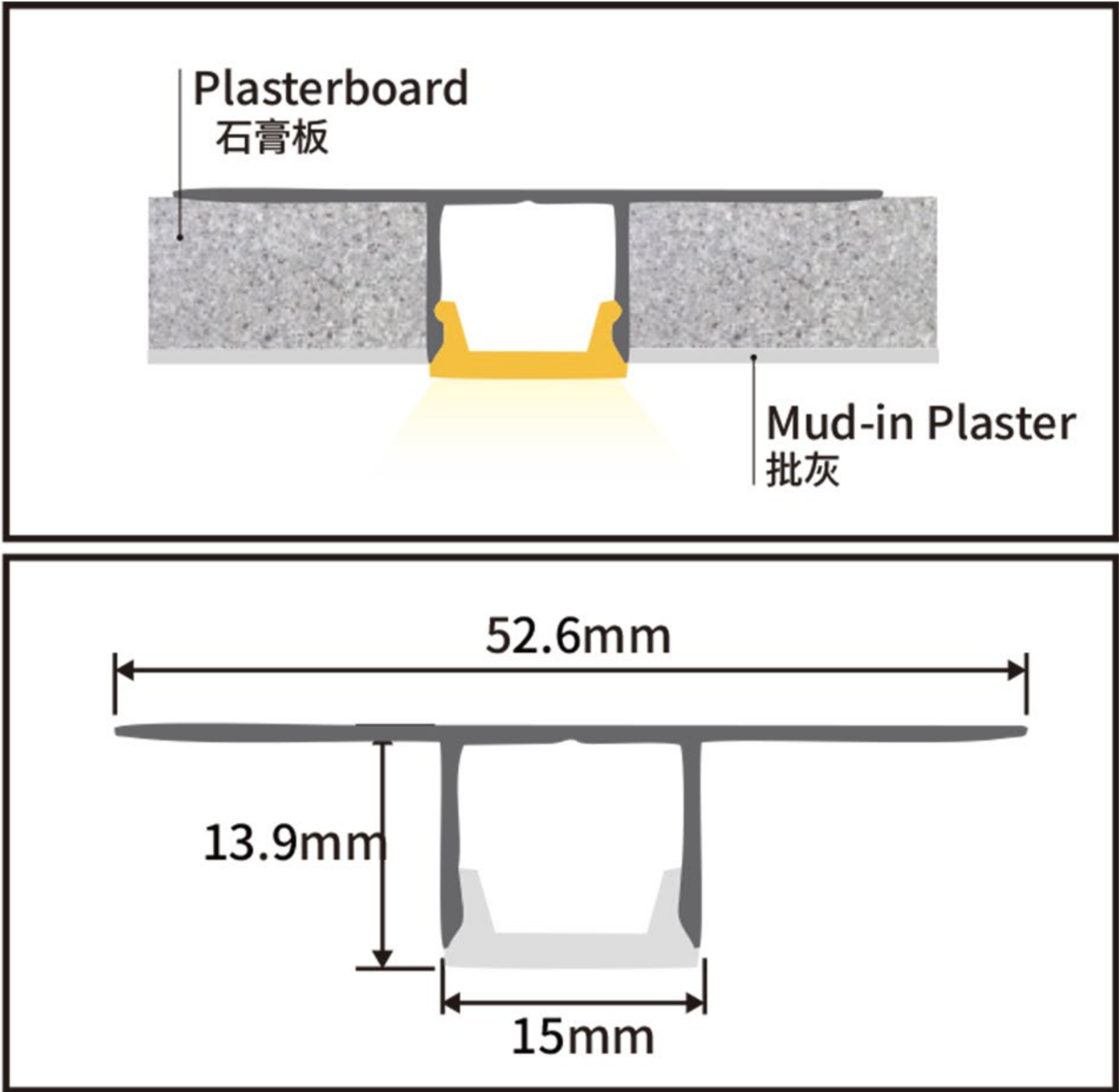
LFAPSL-DW-52.6X13.9X15
