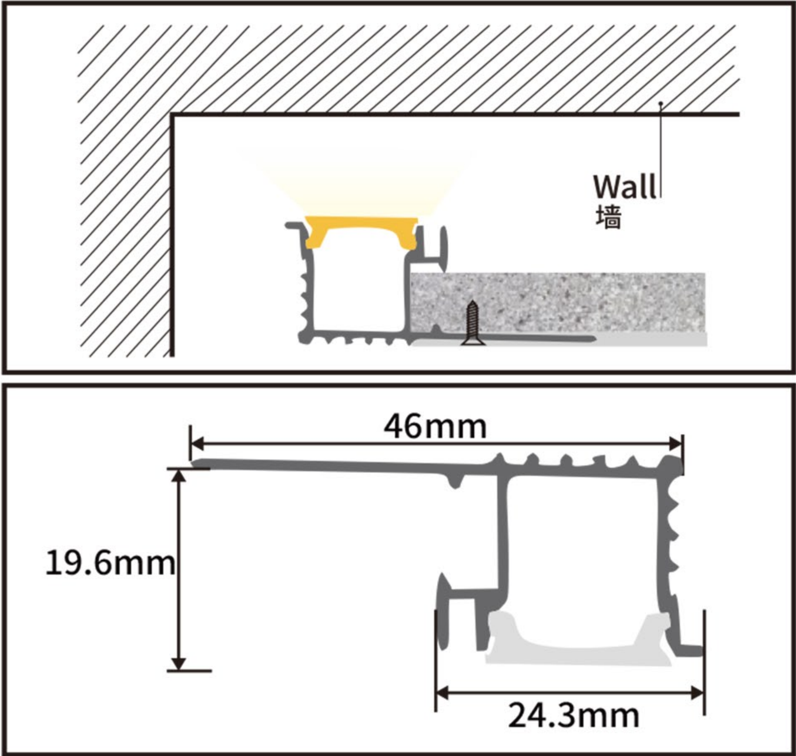
LFAPSL-SWL-46X19.6X24.3
