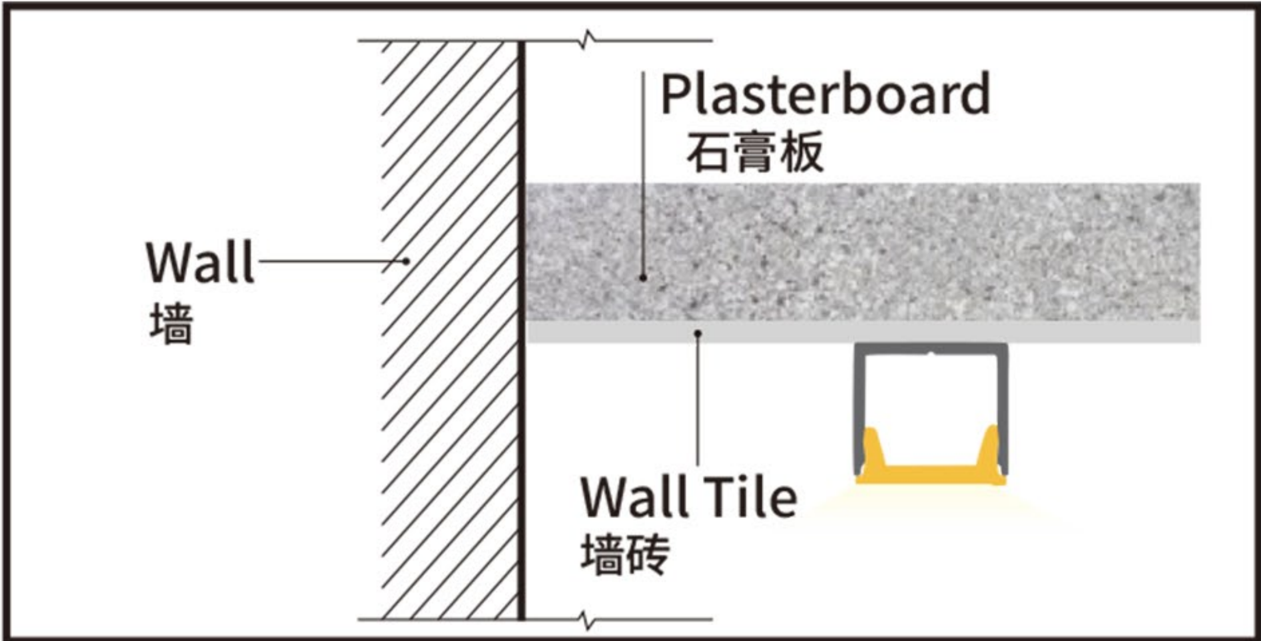
LFAPSL-NW-15X11X12.8
