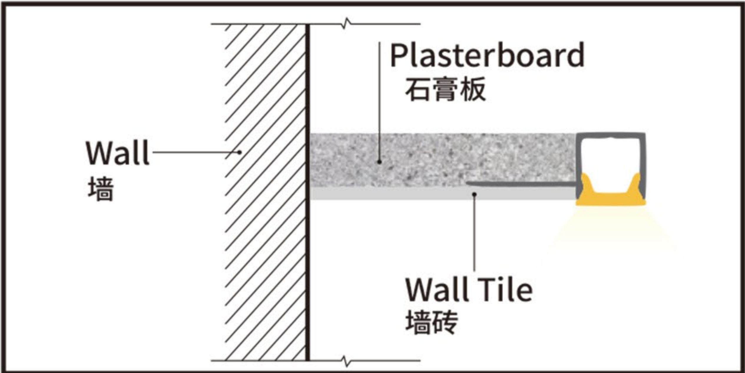
LFAPSL-SWL-32X13X13
