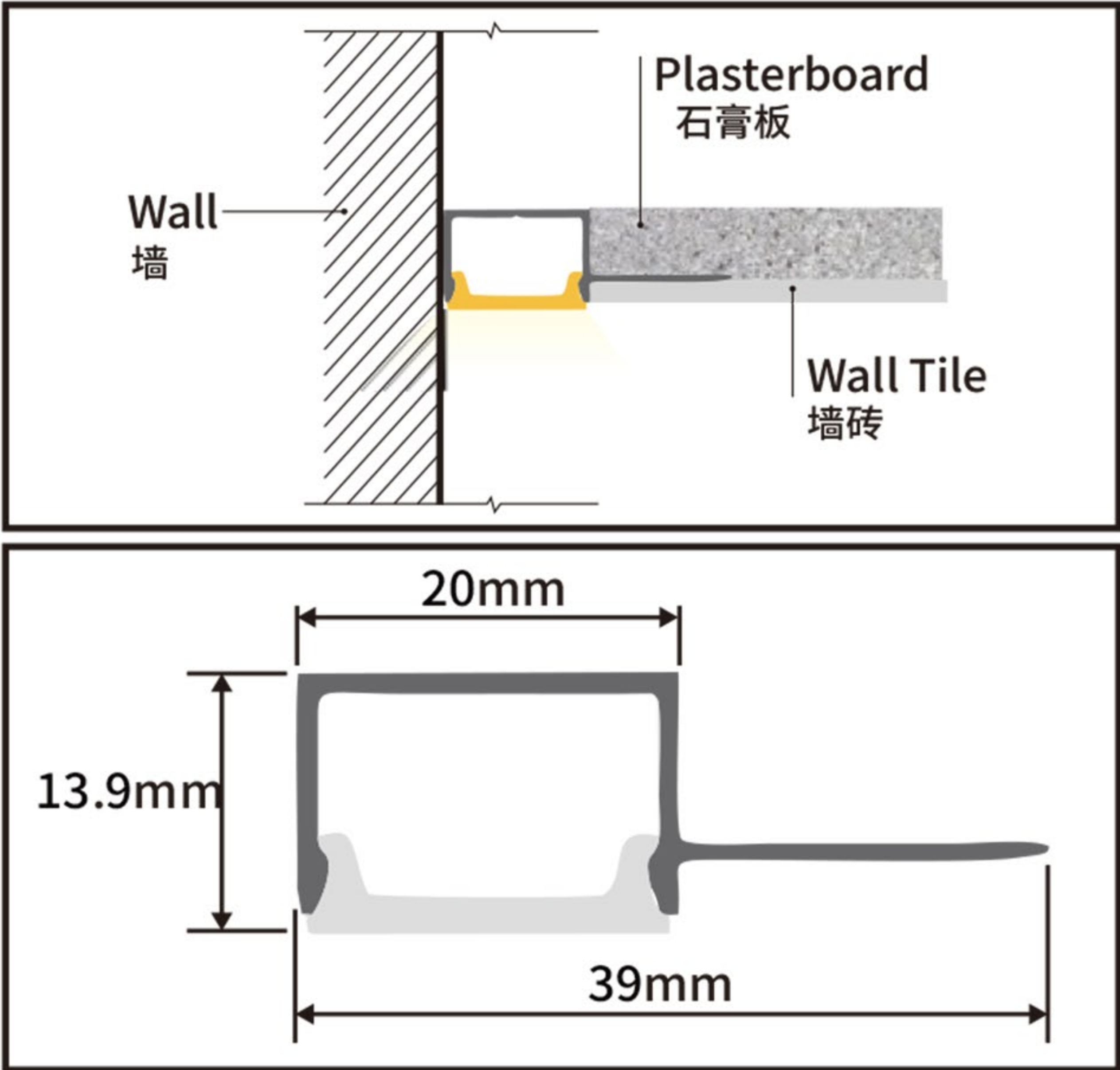
LFAPSL-SWL-39X13.9X20
