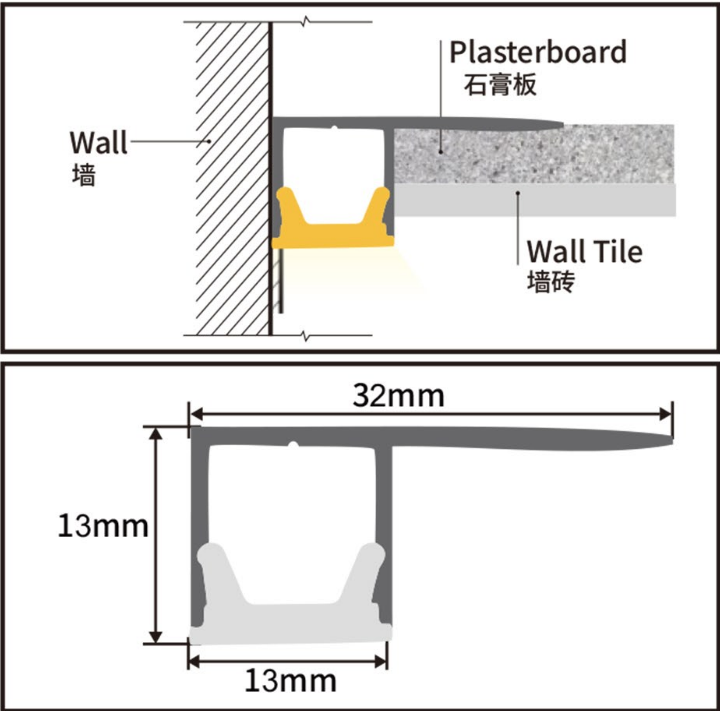
LFAPSL-SWR-32X13X13
